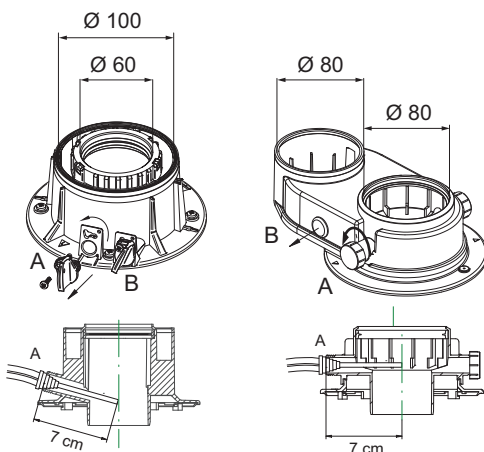
Fig.35 Punto de medición de los gases de combustión según accesorio de conexión a caldera
