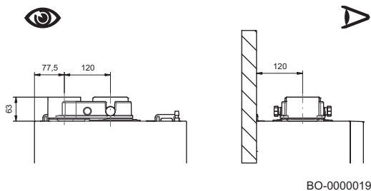
Fig.22 Tipo de aspiración/evacuación desdoblados
