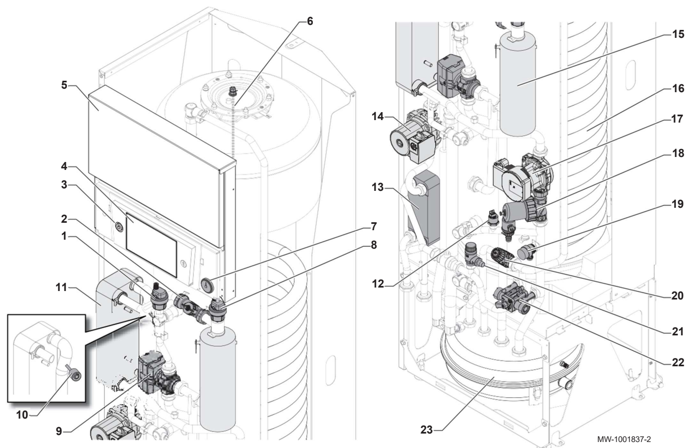
Fig.11 MIC V200 R32 con opción de circuito solar
