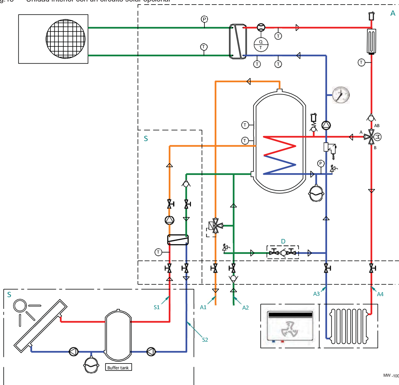
Fig.18 Unidad interior con un circuito solar opcional
